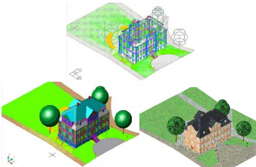
Abb. 10: Datenmodellierung (oben) und Rendering (links) der Landdrostei Pinneberg in AutoCAD (Farbwahl zur Übersichtlichkeit und Trennung der Objektklassen), gerendertes Modell mit Materialzuweisung (rechts)
